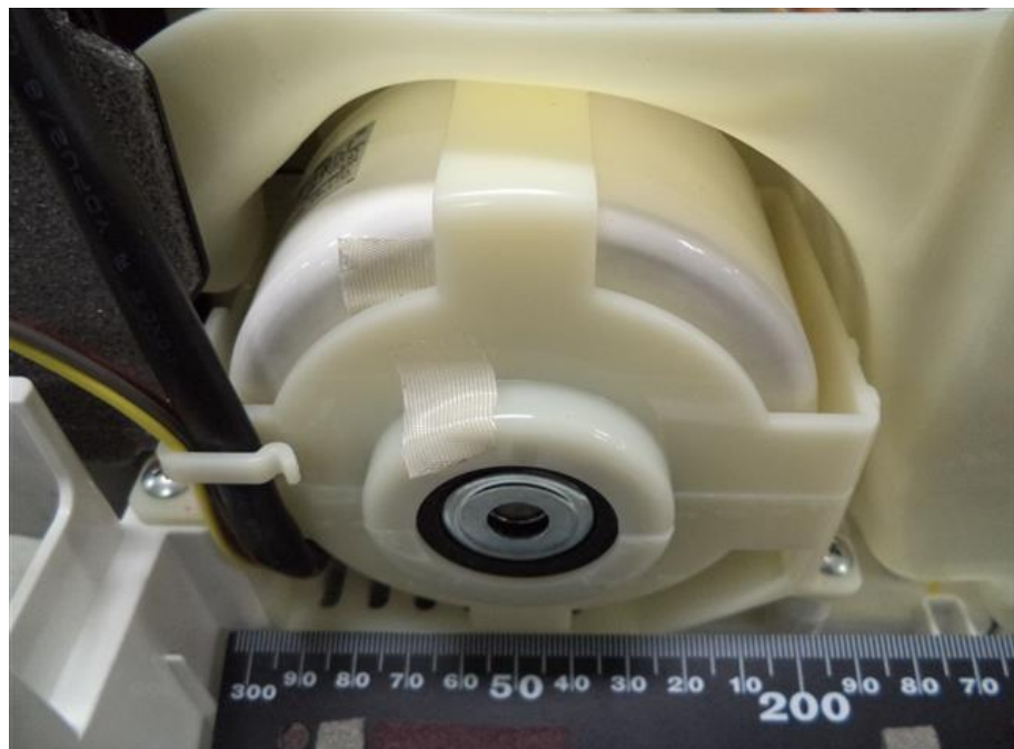
116. RAS-B16PKVSG-E, Indoor fan motor
