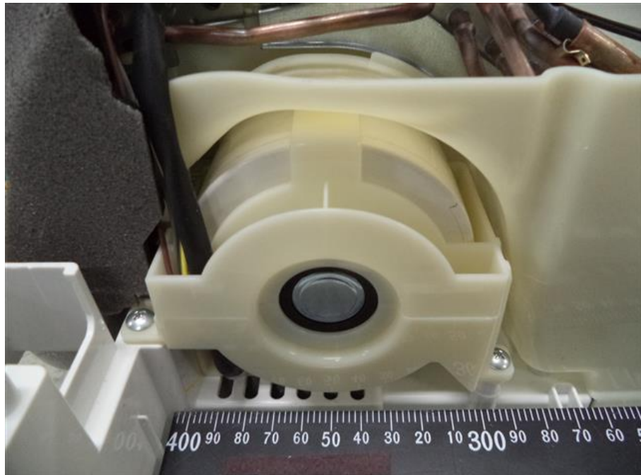
70. RAS-B07BKVG-E, Indoor fan motor
