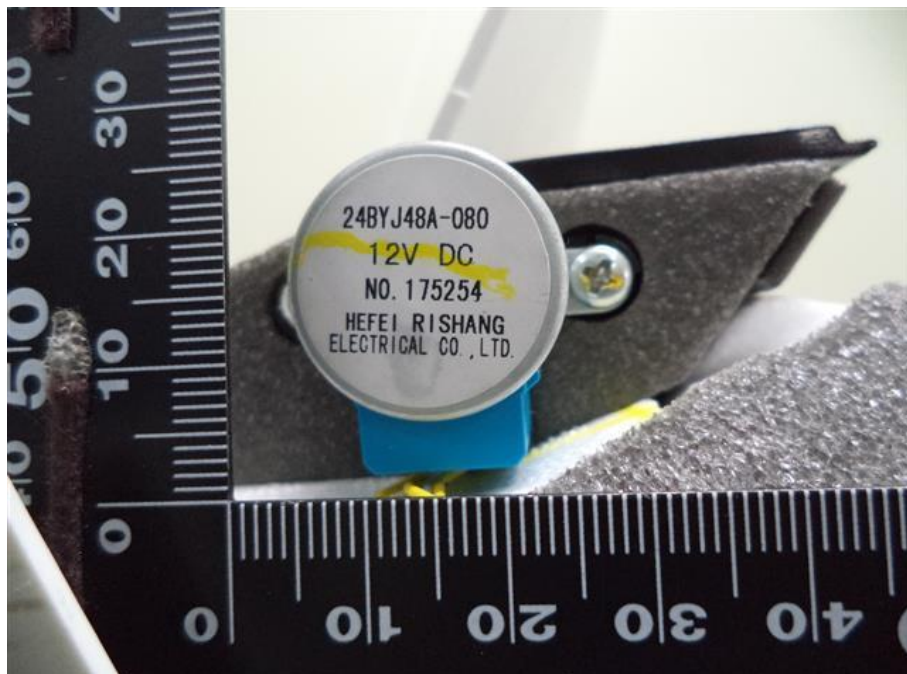
18. RAS-B10PKVSG-E, Louver motor (Vertical)
